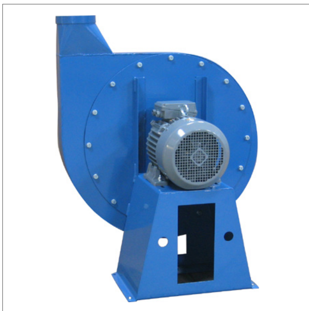
HV - Fan for clean air
